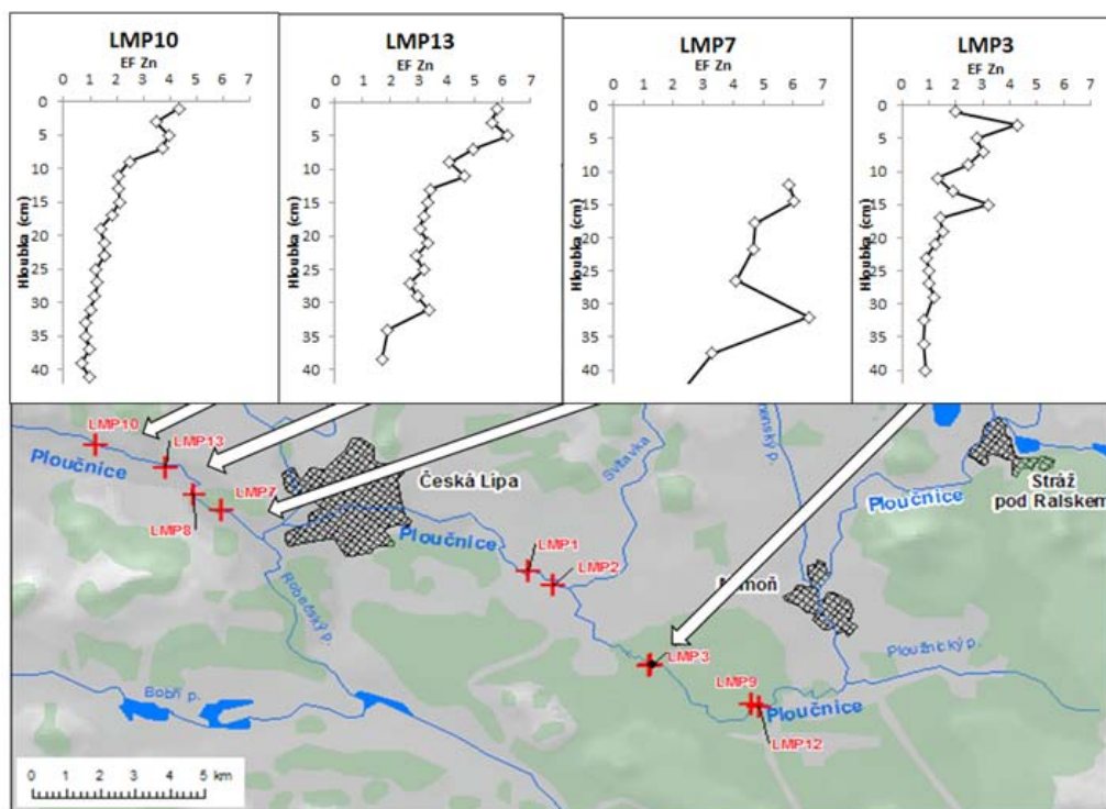
Obr. 12 Nárůst faktoru nabohacení Zn v hlubkových profilech LMP7, LMP13, LMP10 v oblasti mezi Českou Lípou a obcí Jezvė, ve srovnání s hlubkovým profilem LMP3 z oblasti mezi Mimoňí a Českou Lípou
