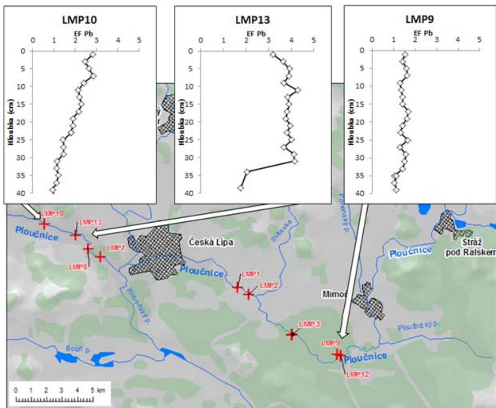
Obr. 11 Nárůst faktoru nabohacení Pb v hlubkových profilech LMP13, LMP10 z oblasti mezi Českou Lípou a obcí Jezvė, ve srovnání s hlubkovým profilem LMP9 z oblasti mezi Mimoňí a Českou Lípou
